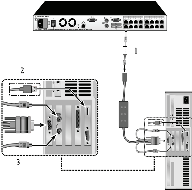
그림 2-11. SIP 연결
